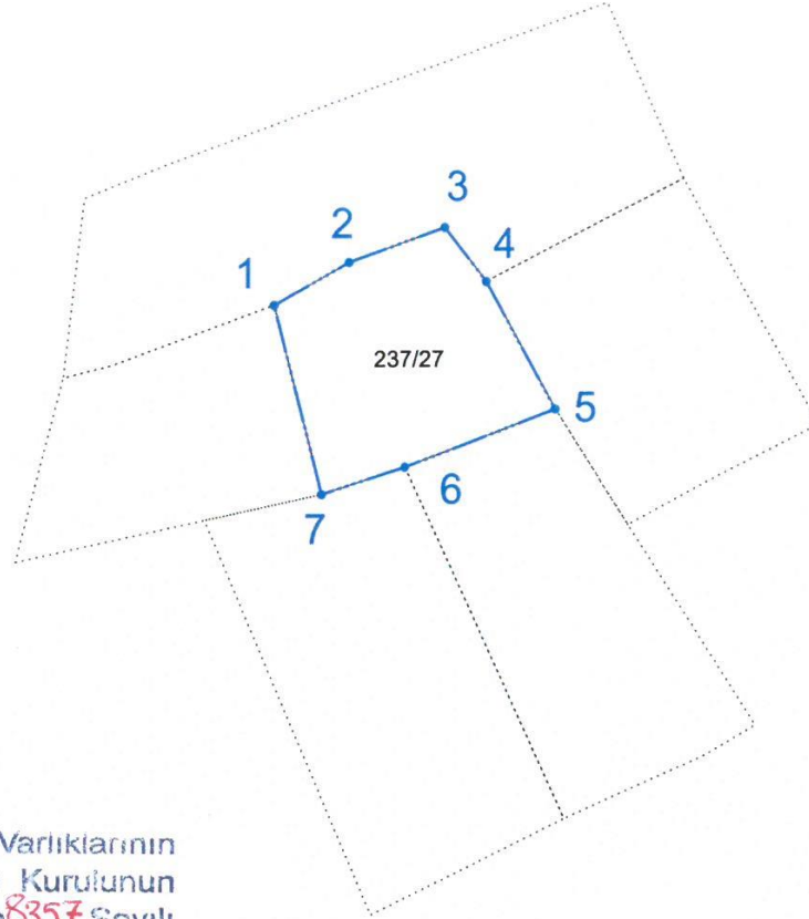
ITRF96 UTM 3 Derecelik Koordinatlar
